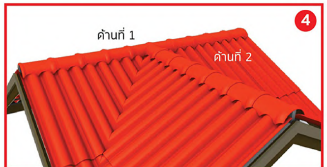
การติดตั้งครอบสันหลังคาตัวสุดท้ายของด้านที่ 2 ให้แนบสนิท และสวยงาม
