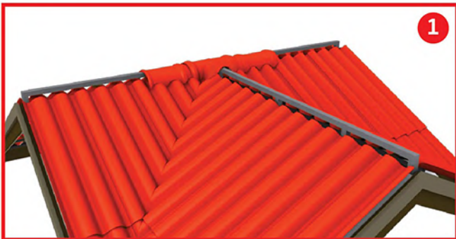
เริ่มจากการวางครอบสันหลังคาตัวแรกให้ตรงตำแหน่งที่แนวสันหลังคา อีกด้านหนึ่งที่มาบรรจบ แล้วยึดด้วยคัลเลอร์สกรู/สกรูคลาส 3
