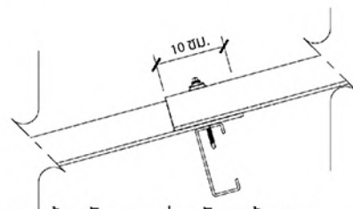
ภาพที่ 2: แนวการซ้อนทับของแผ่นหลังคาด้านยาว ที่มีการซ้อนทับ 10 ซม.
