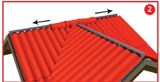
การติดตั้งครอบสันหลังคา ให้ติดตั้งออกไปทางด้านซ้าย และขวา จนสุดแนวสันหลังคาทั้ง 2 ด้าน
