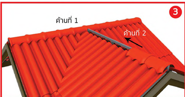
การวางครอบสันหลังคา ด้านที่ 2 (ตามรูป) ให้เริ่มจากด้านป็นลมเข้ามา บรรจบกับแนวสันหลังคา ด้านที่ 1
