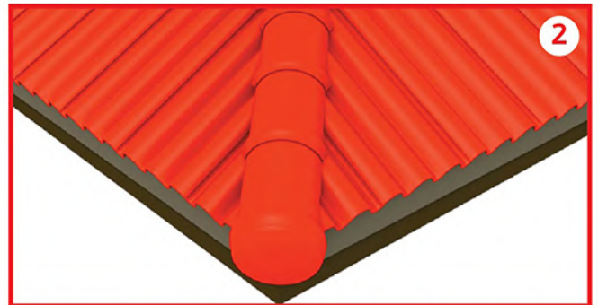
ให้เริ่มวางครอบปิดชายสันตะเข้ลงบนครอบสันตะเข้ไตรลอน และทำการยึดด้วยคัลเลอร์สกรู / สกรูคลาส 3
