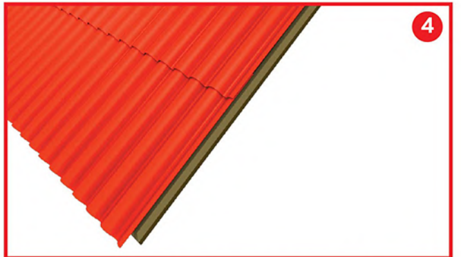
แนวแผ่นหลังคาที่ติดกับป็นลม ให้เป็นลอนหงายเสมอกับไม้ป็นลม เมื่อต้องใช้ครอบตกแต่ง และให้เป็นลอนคว่ำเมื่อไม่ใช้ครอบตกแต่ง
